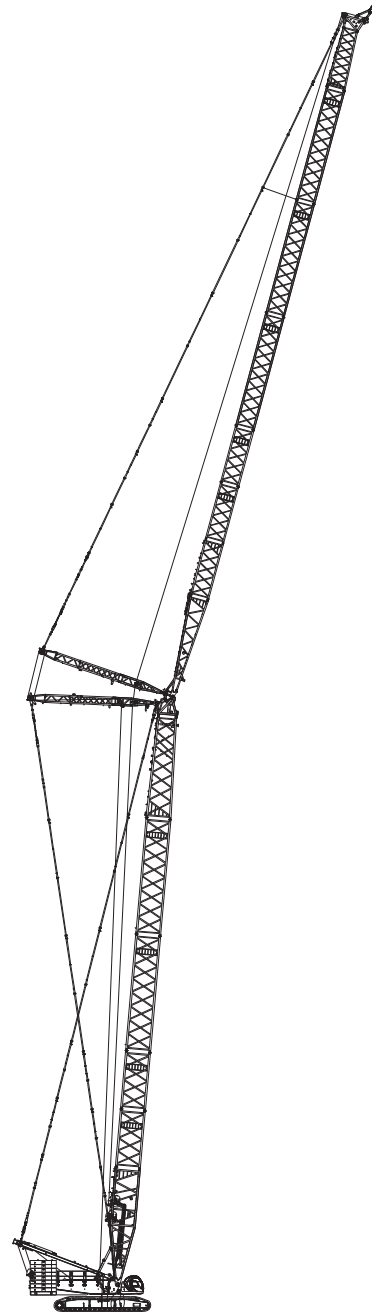
主臂 + 变幅副臂LJ60+72
