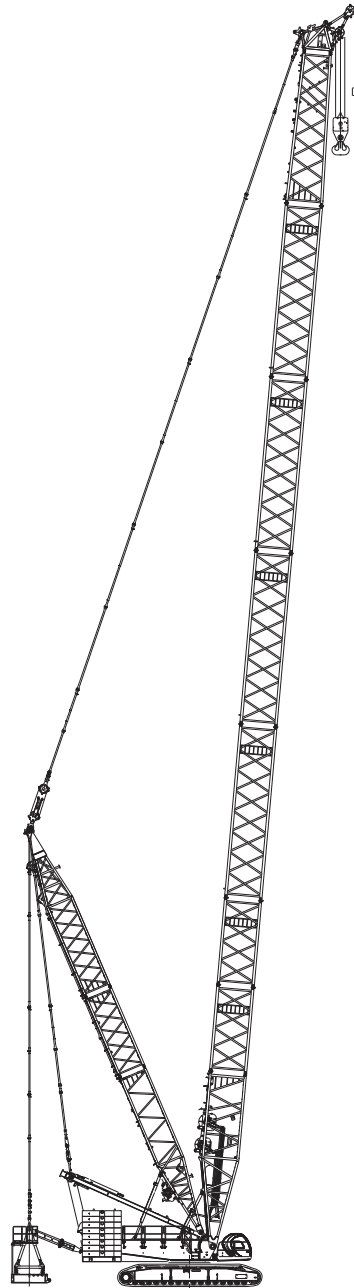
主臂超起工况HDB84m
